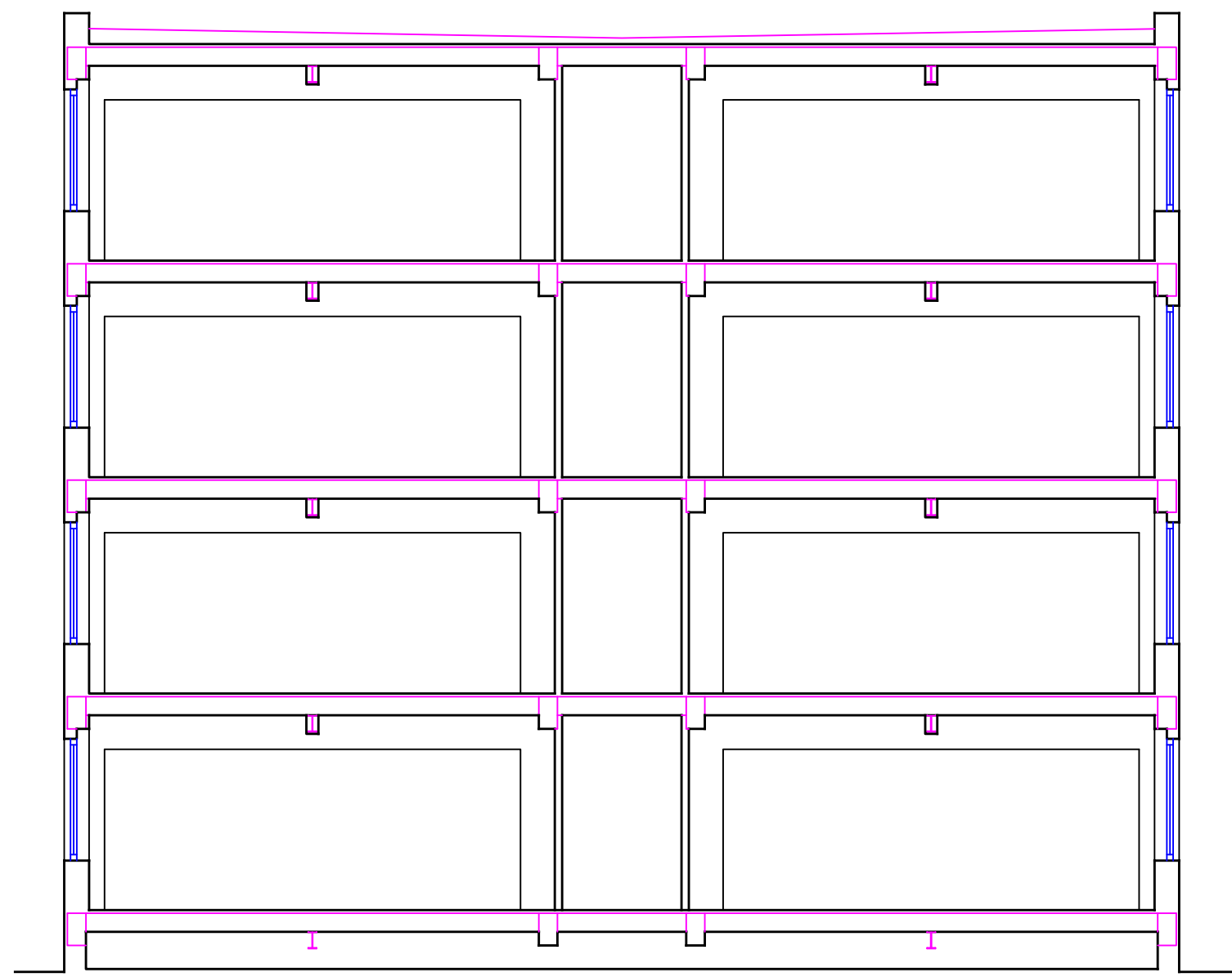
SECCIÓN 1
