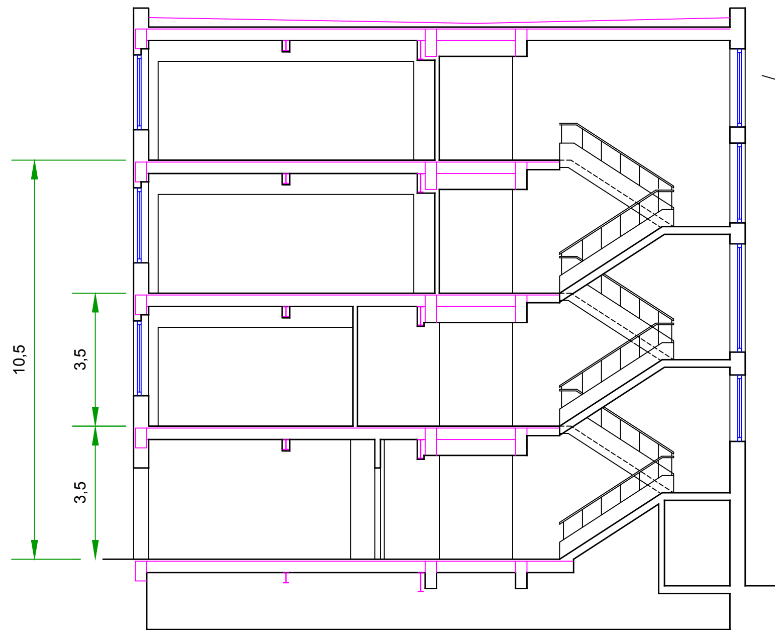
SECCIÓN 2
