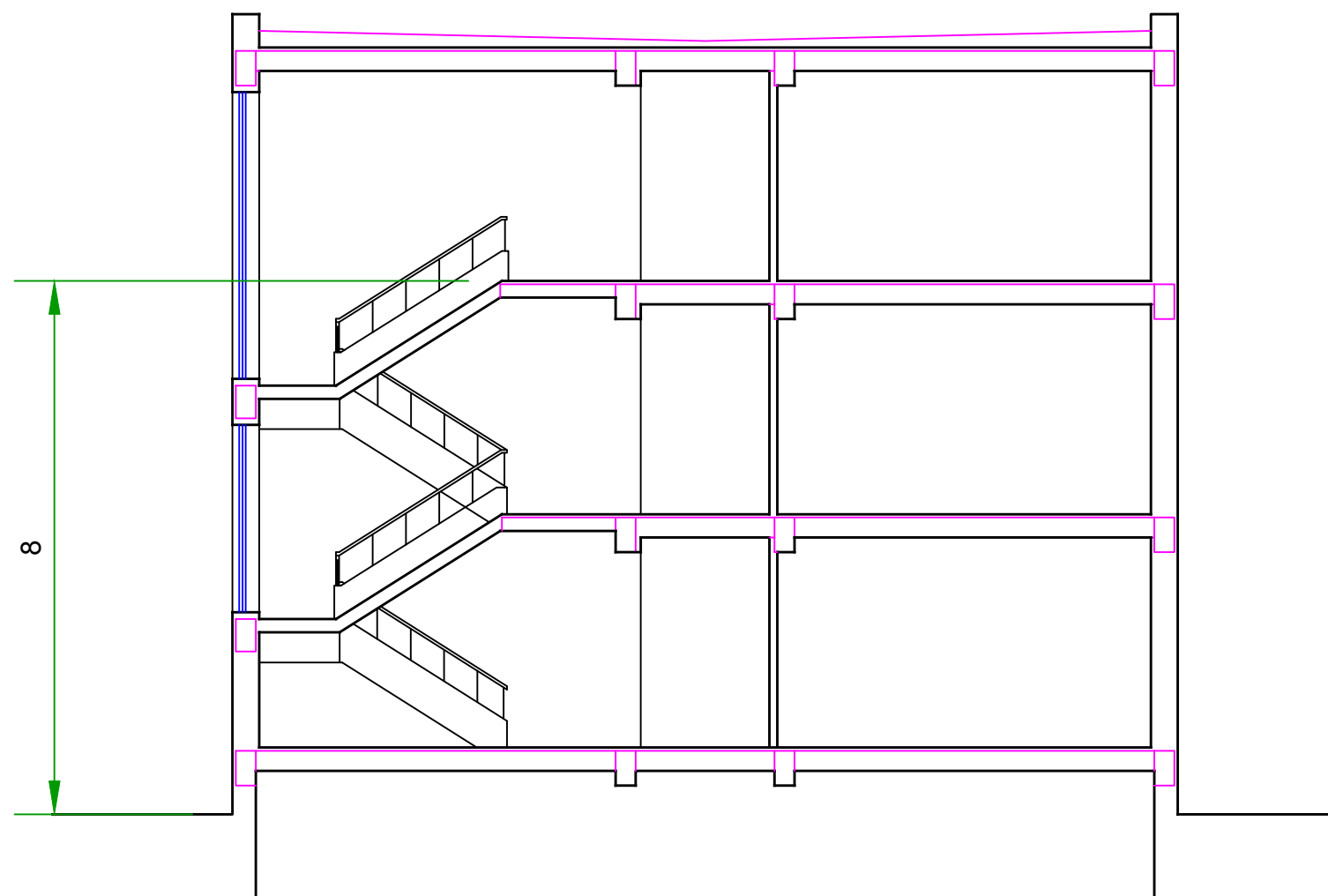
SECCIÓN 3
